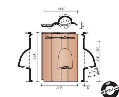
8958 Kabeldoorvoerpan met neopreen ring
