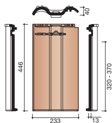
8050 Pan met dubbele wel
