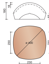
5140 Nr 13: Vorstenhoed 3 x 1200
