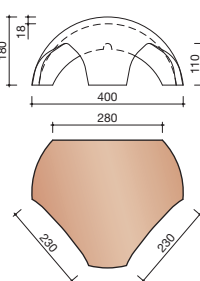
5520 Nr 3: Vorstenhoed 1 x 1200 en 2 x 3100
