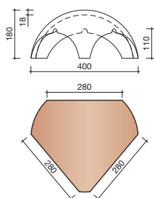
5580 Nr. 9: vorstenhoed 3 x 1200
