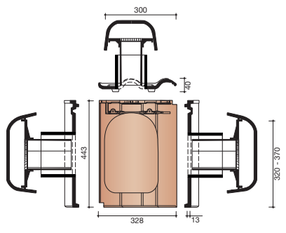
8728 Dakdoorvoer incl. aansl. Ø 125 mm
