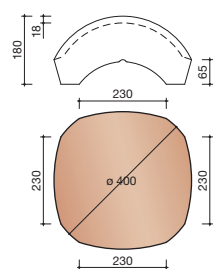
5540 Nr. 5: vorstenhoed 4 x 1200
