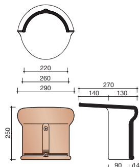
1215 Halfronde begin-/eindvorst vario
